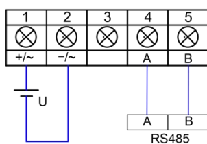
выход RS485
