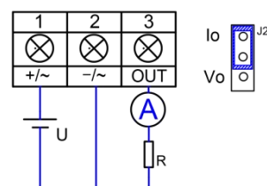
выход 4-20 мА
